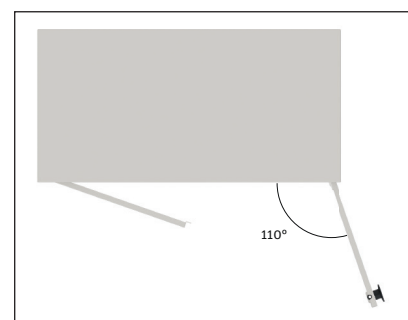
Angle d'ouverture de la porte battante
